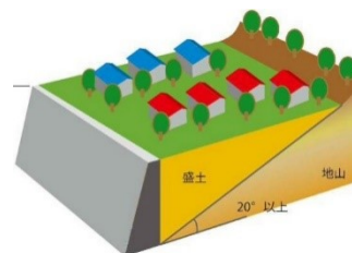
(盛り土造成地)
